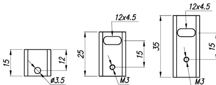
HRU-20/15 16 K/W
