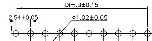
P.C.B. Layout
