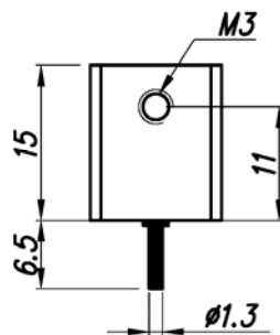
HR-95/15+PIN SOT32 38,5 K/W
